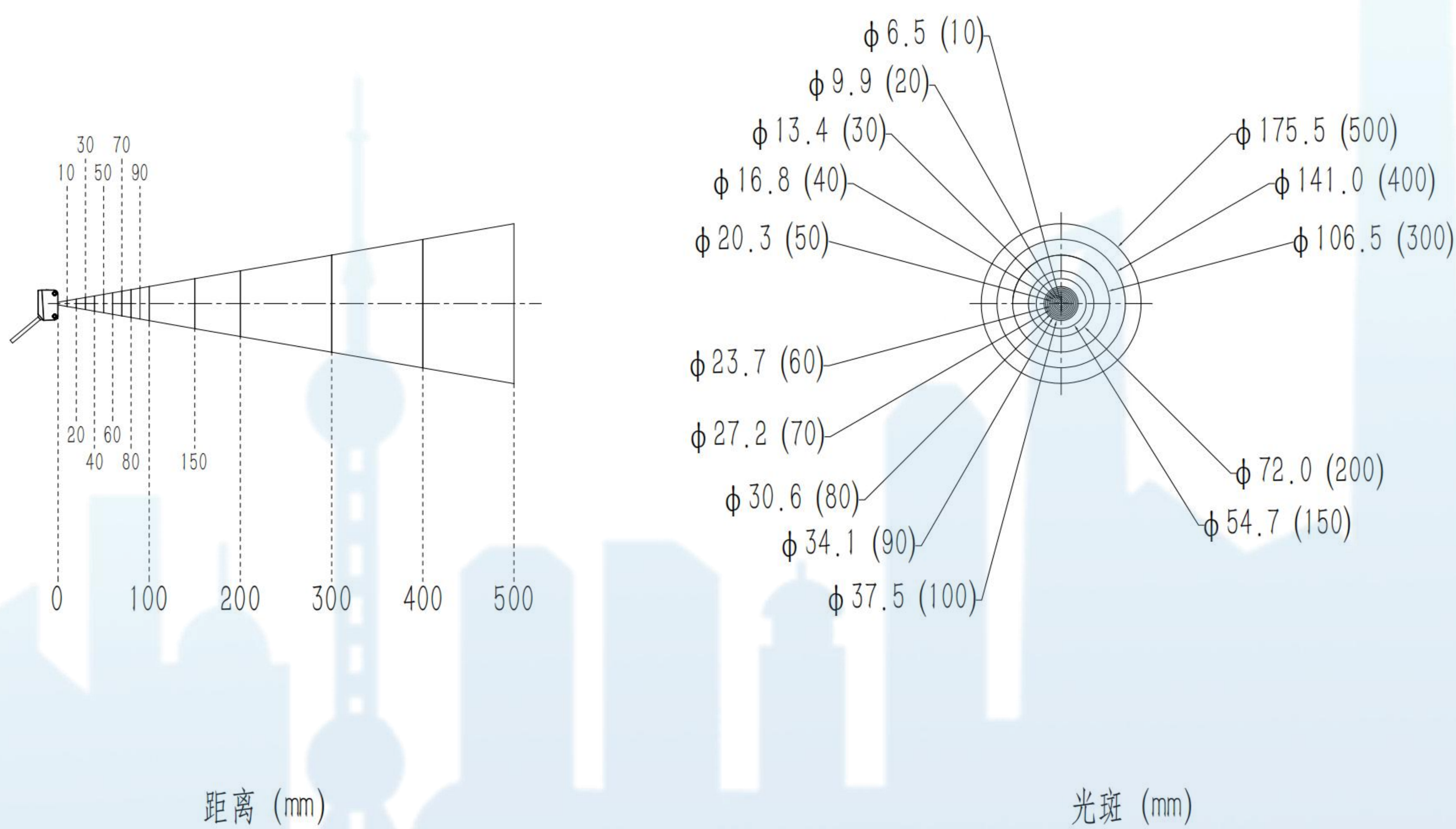
PS04系列光斑图
