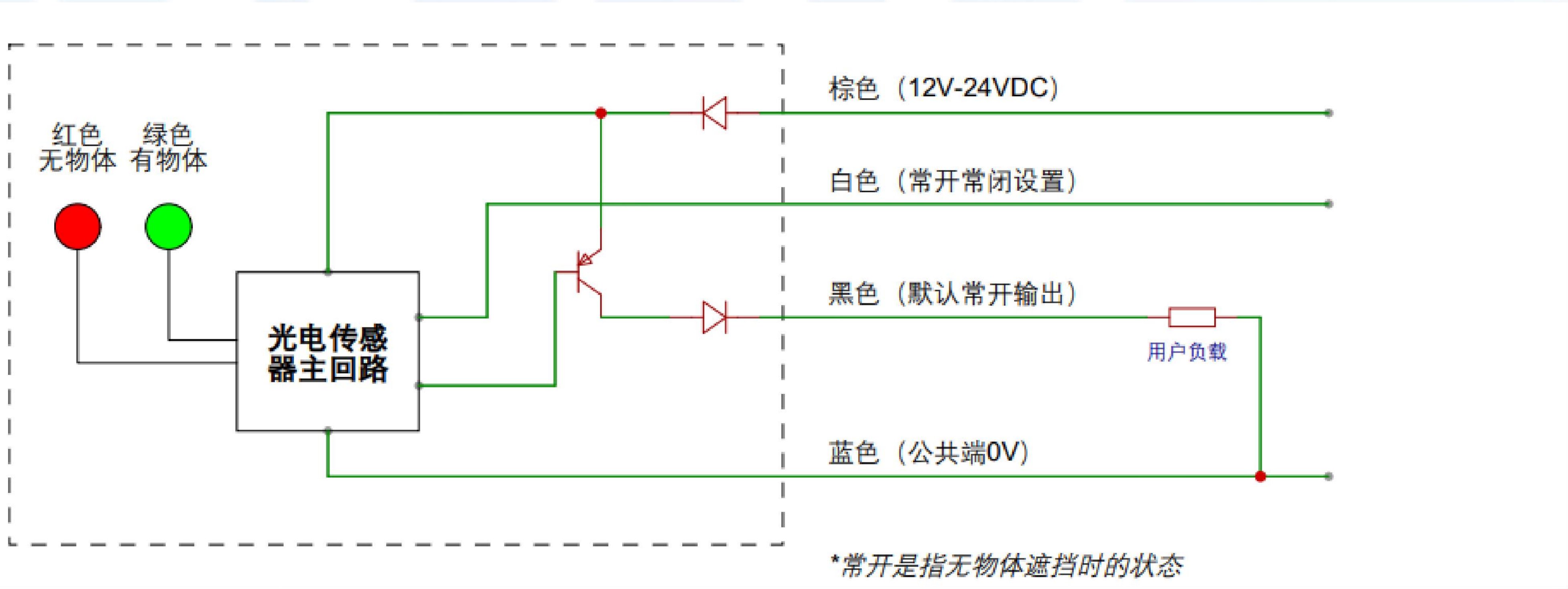
PNP集电极开路输出示意图（仅供参考）
