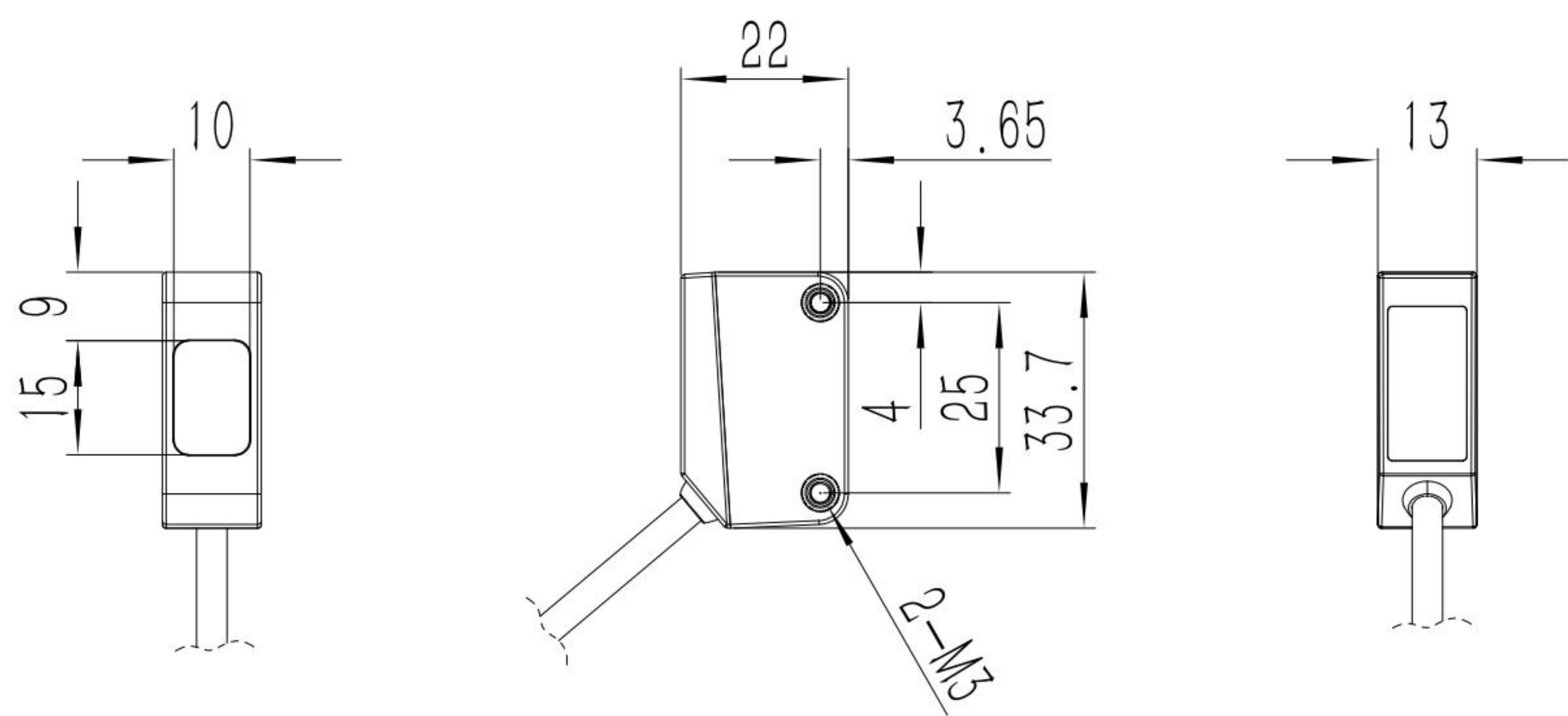
PS04系列尺寸图
