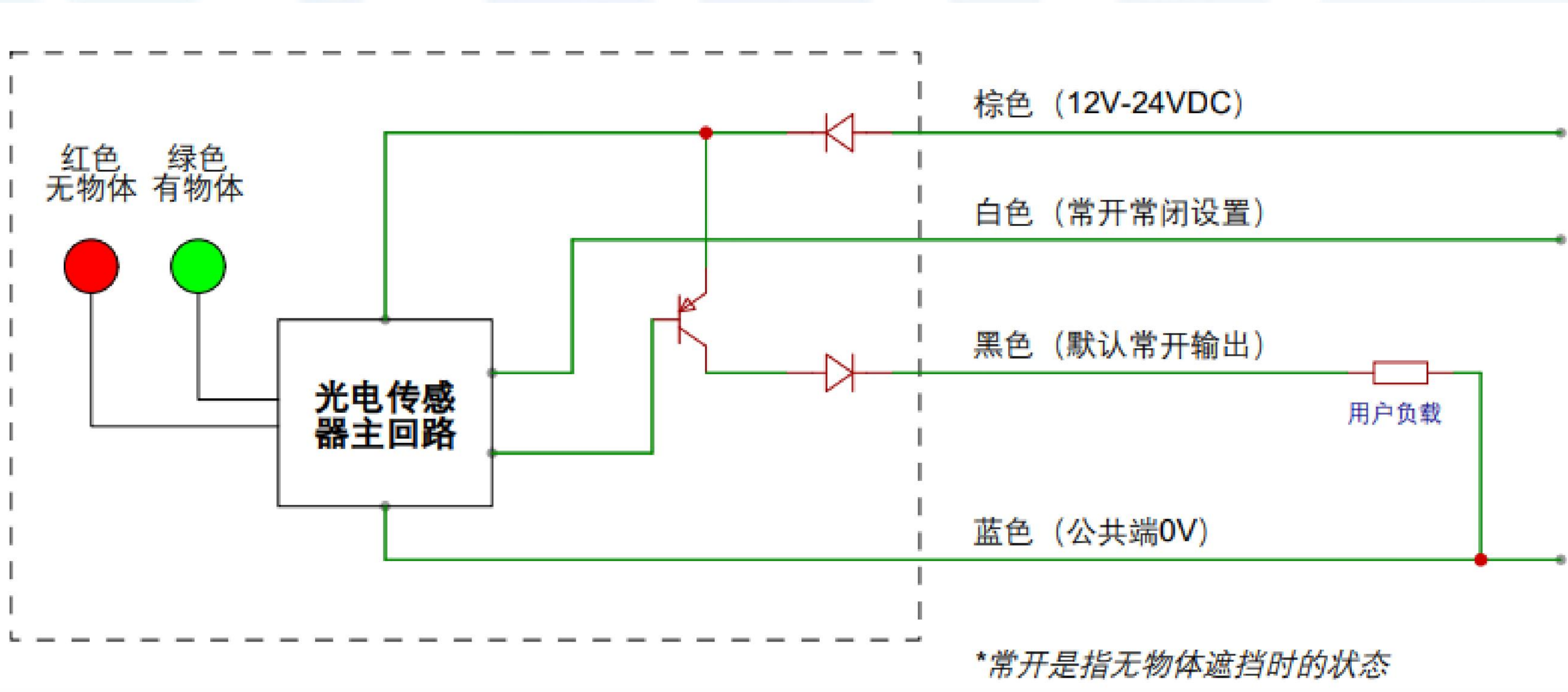
PNP集电极开路输出示意图（仅供参考）
