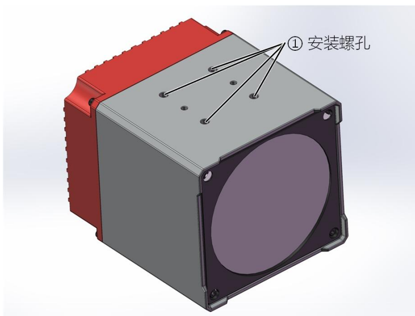
图 4.1: 无配件安装
