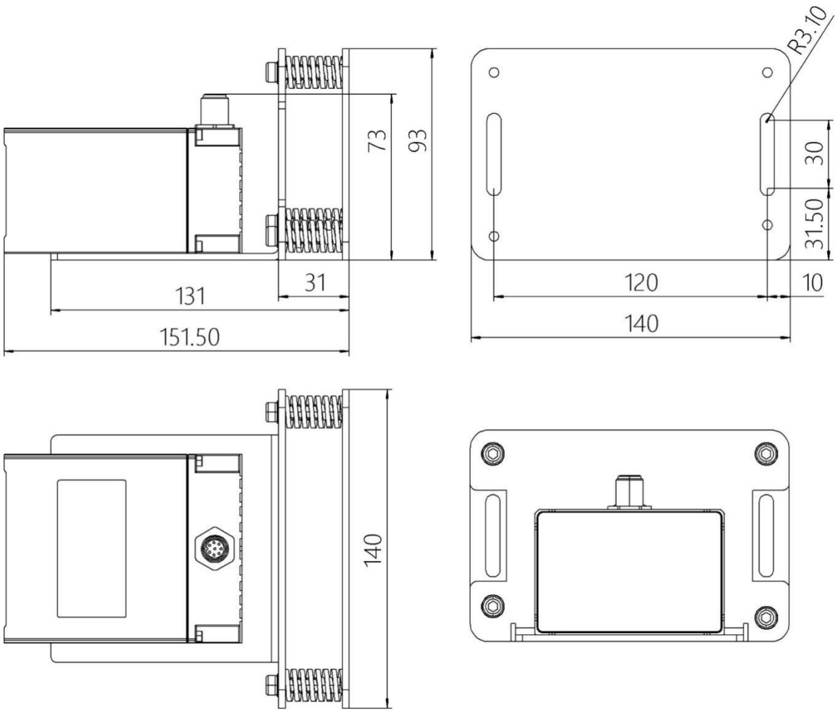
图 3.2: 支架组装尺寸图 (单位: mm)
