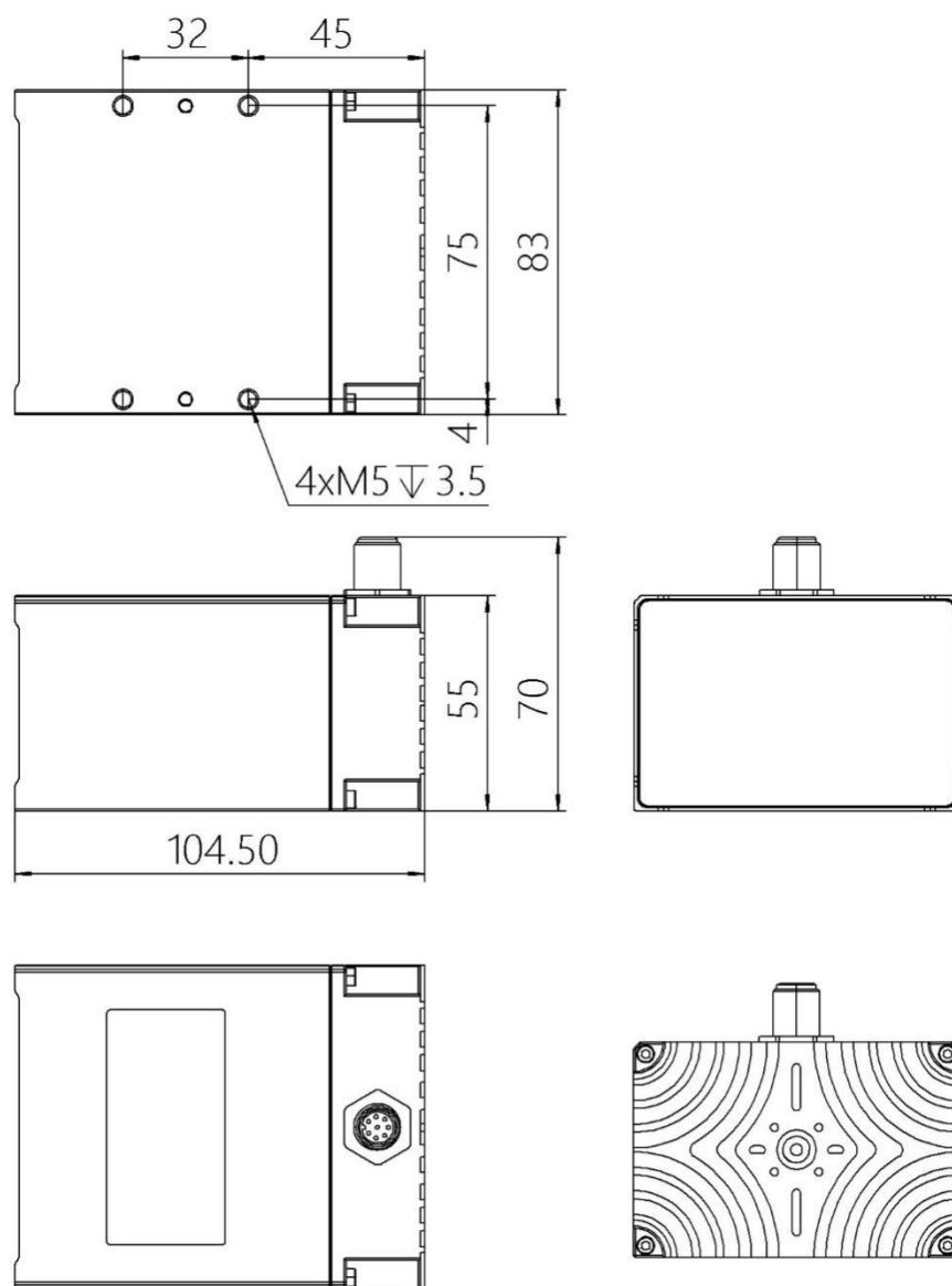
图 3.1: 传感器尺寸图 (单位: mm)
