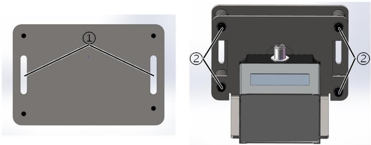
图 4.2: 可调支架安装
