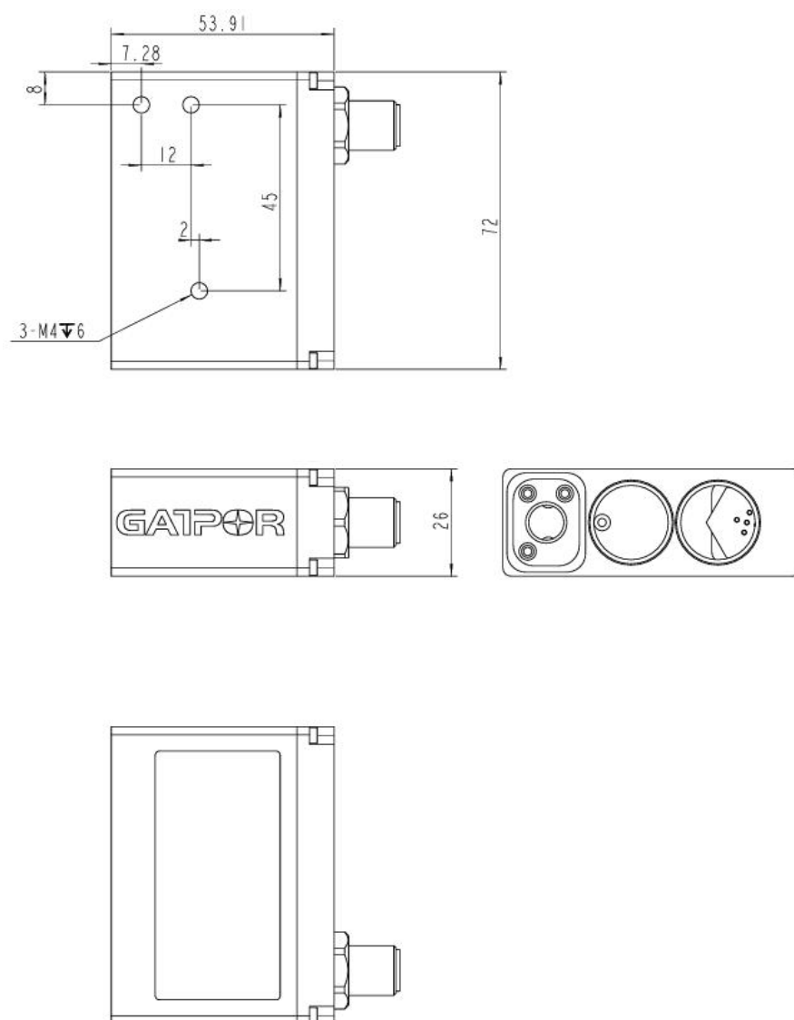
图 3.1: 传感器尺寸图 (单位: mm)
