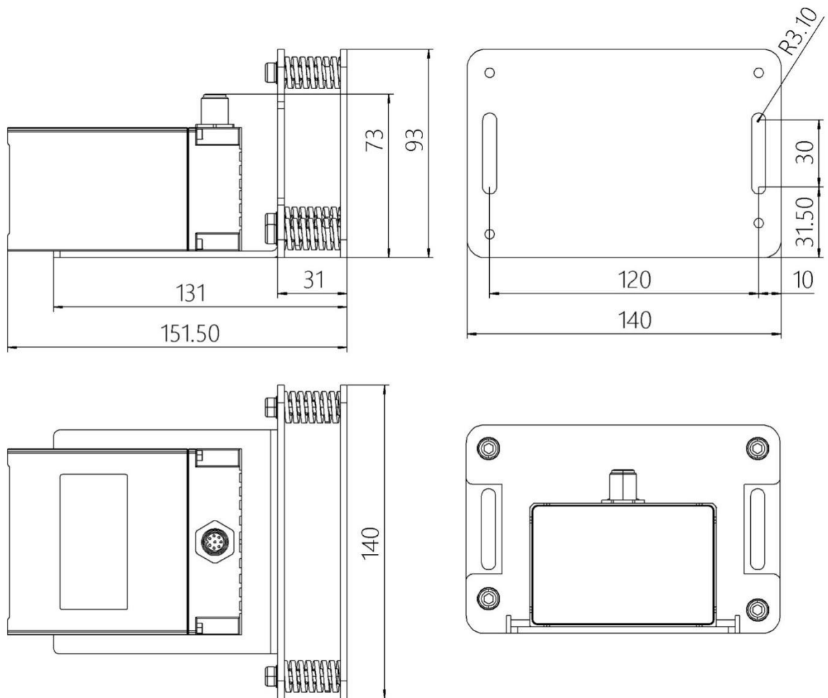
图 3.2: 支架组装尺寸图 (单位: mm)
