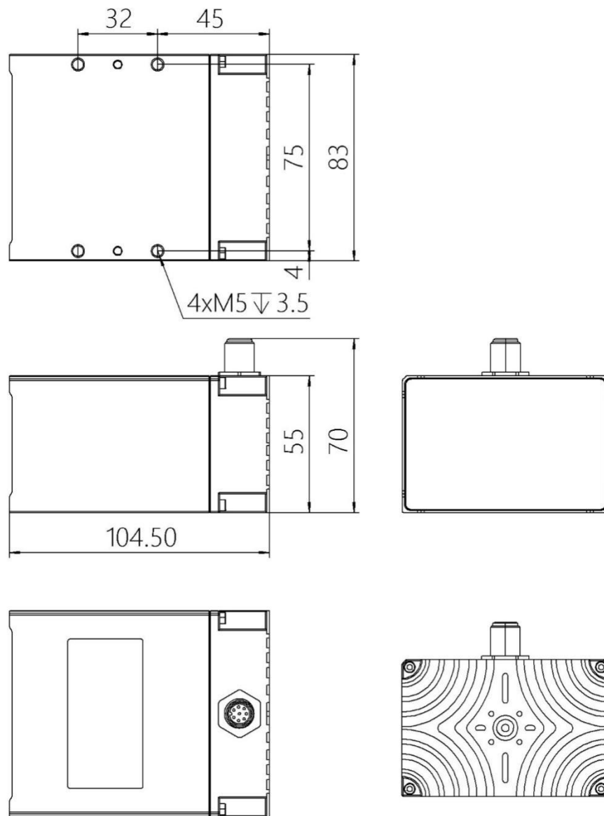
图 3.1: 传感器尺寸图 (单位: mm)
